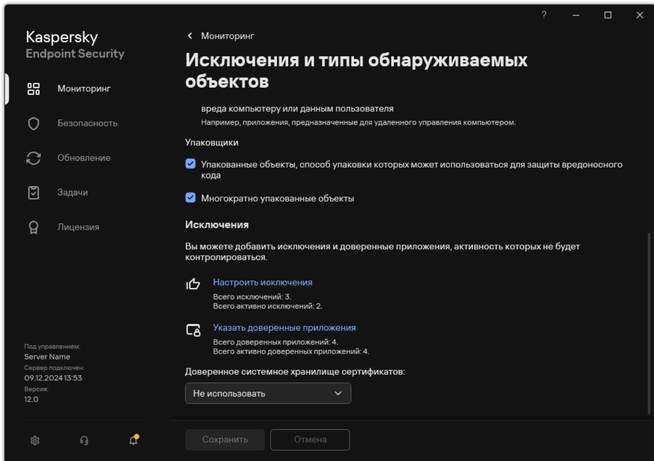
Рисунок 90. Параметры исключений
