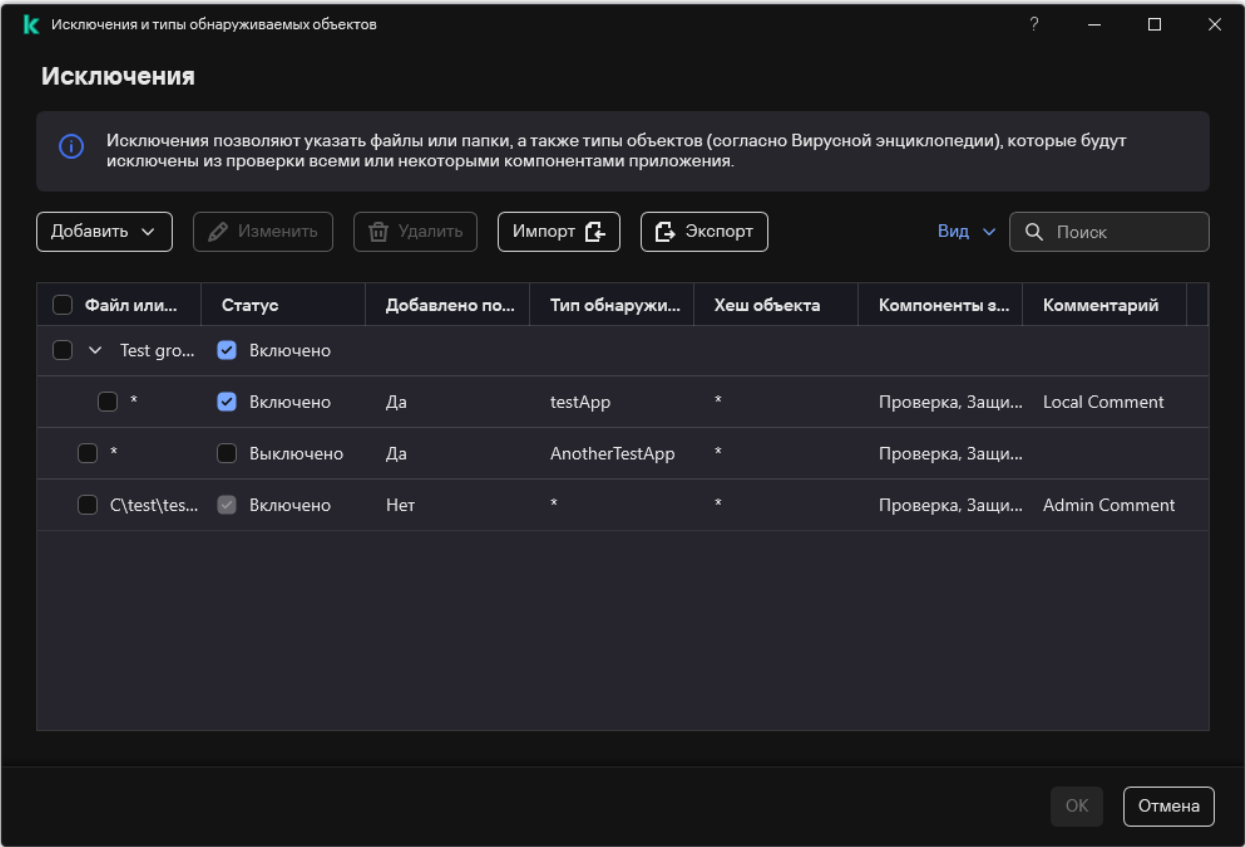
Рисунок 88. Список исключений
