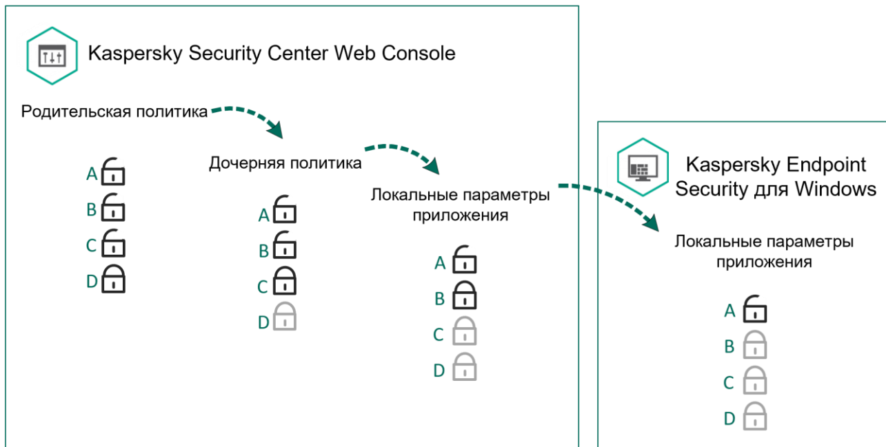
Рисунок 10. Наследование параметров
