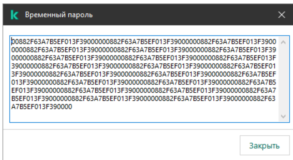
Рисунок 104. Временный пароль
