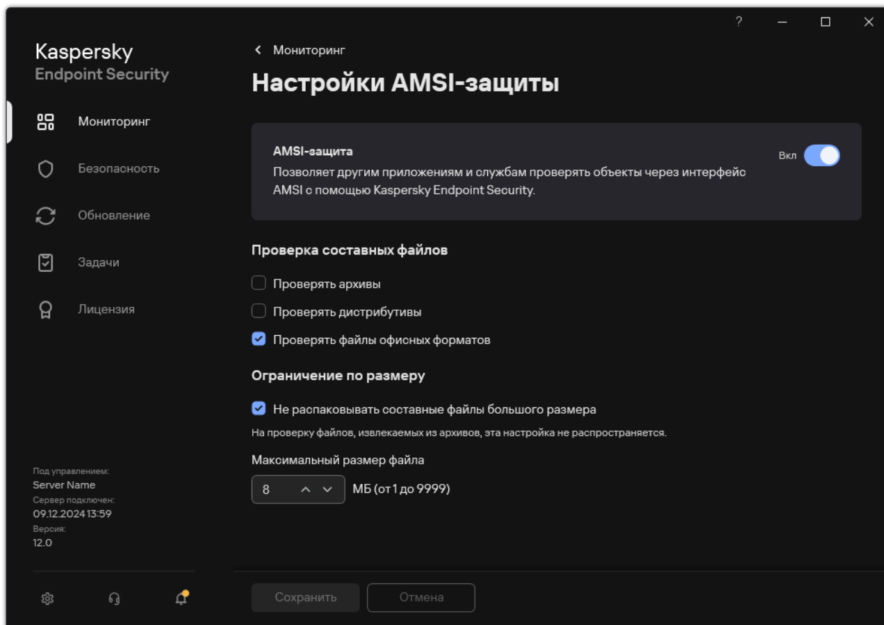
Рисунок 54. Параметры AMSI-защиты
