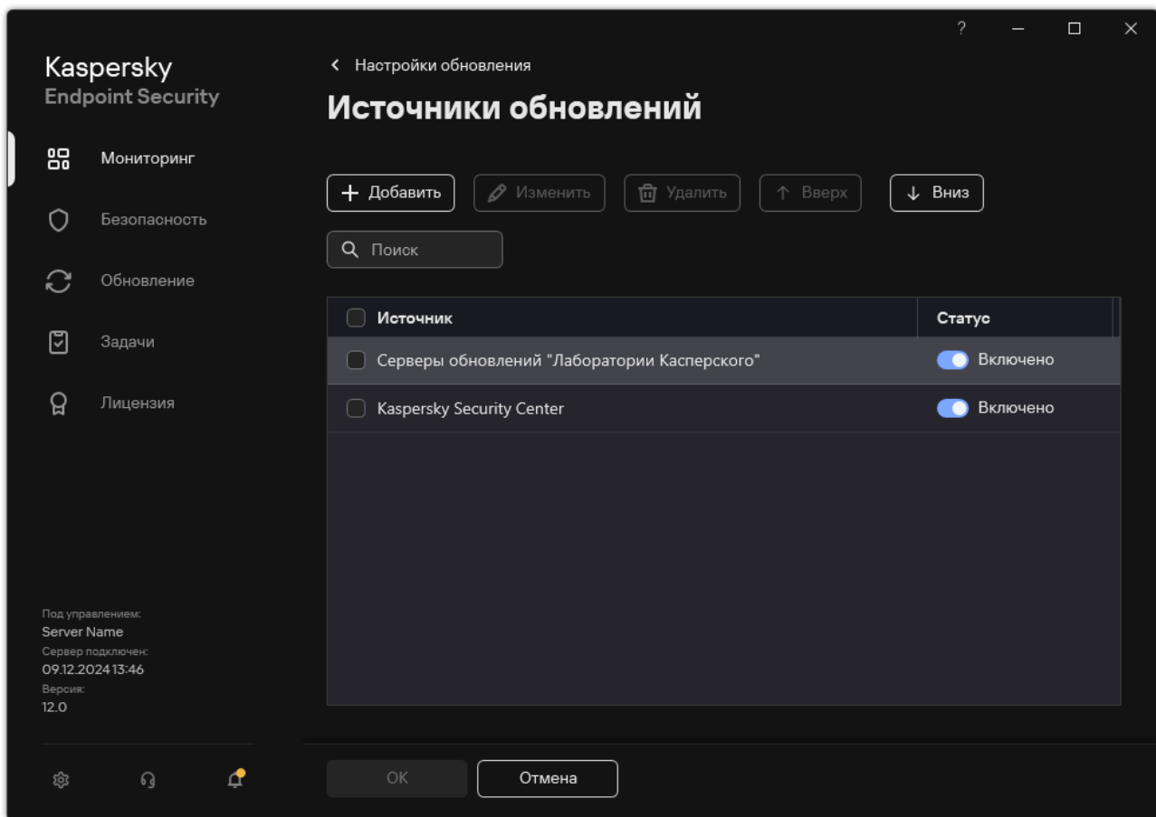
Рисунок 26. Источники обновлений
